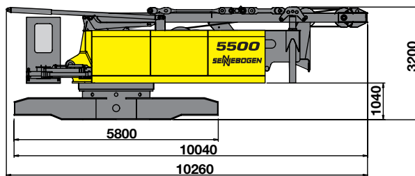
5500 Grundmaschine ohne Fußstück 5500 basic machine without lower boom
