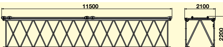
Ausleger - Zwischenstück 11,2 m Typ SH 2027 (mit Abspannung) Boom insert 11.2 m type SH 2027 with pendants
