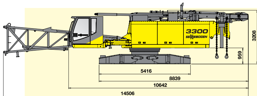
3300 Grundmaschine mit Fußstück 3300 basic machine with lower boom
