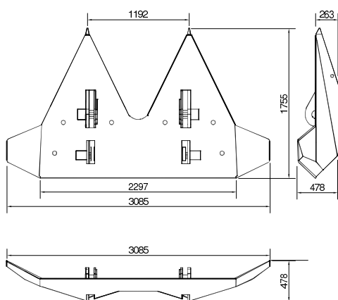
Stevpris
