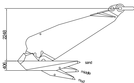
Stevpris
