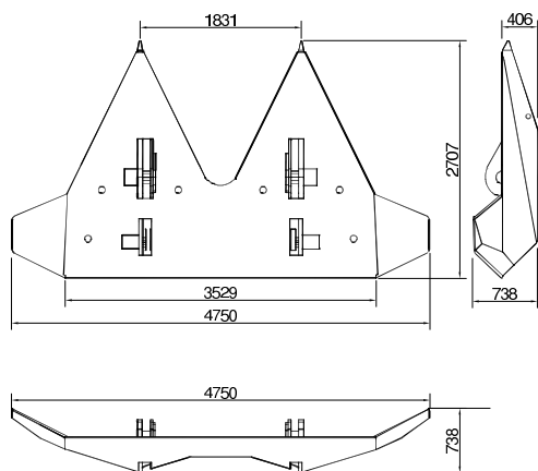
Stevpris
